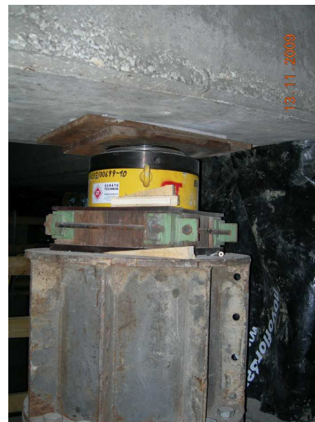
P6) Foto 12 b: maximale Anhebekraft ca. 4.000 KN
